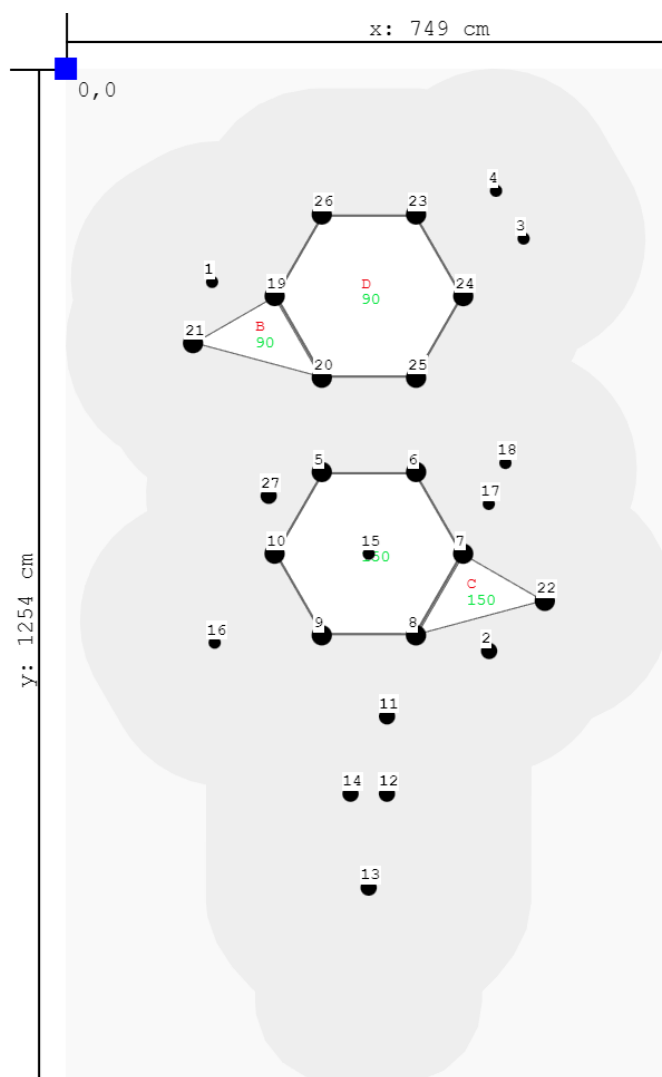
Plattegrond palenplan
