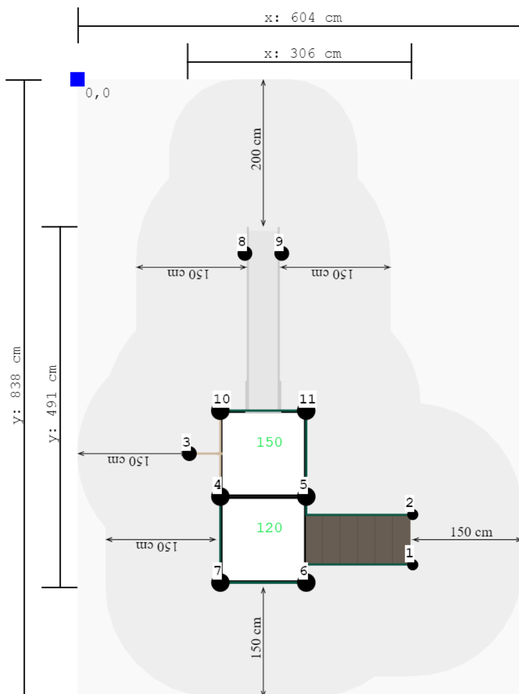
Veiligheidsruimtes
