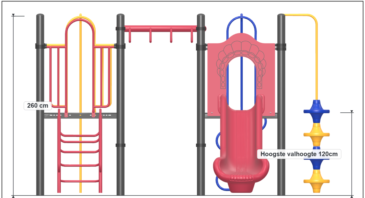
Aanzicht 1
